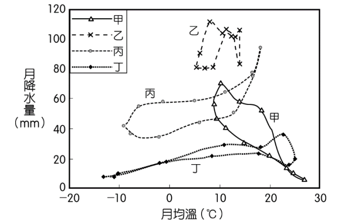
圖 12 溫帶四種氣候分布圖
