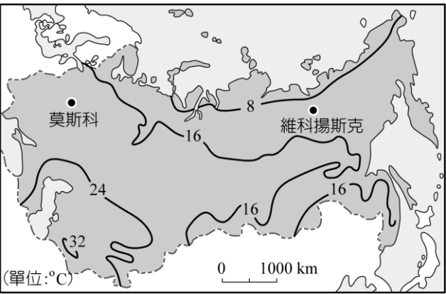
圖 10 獨立國協七月等溫線分布圖
